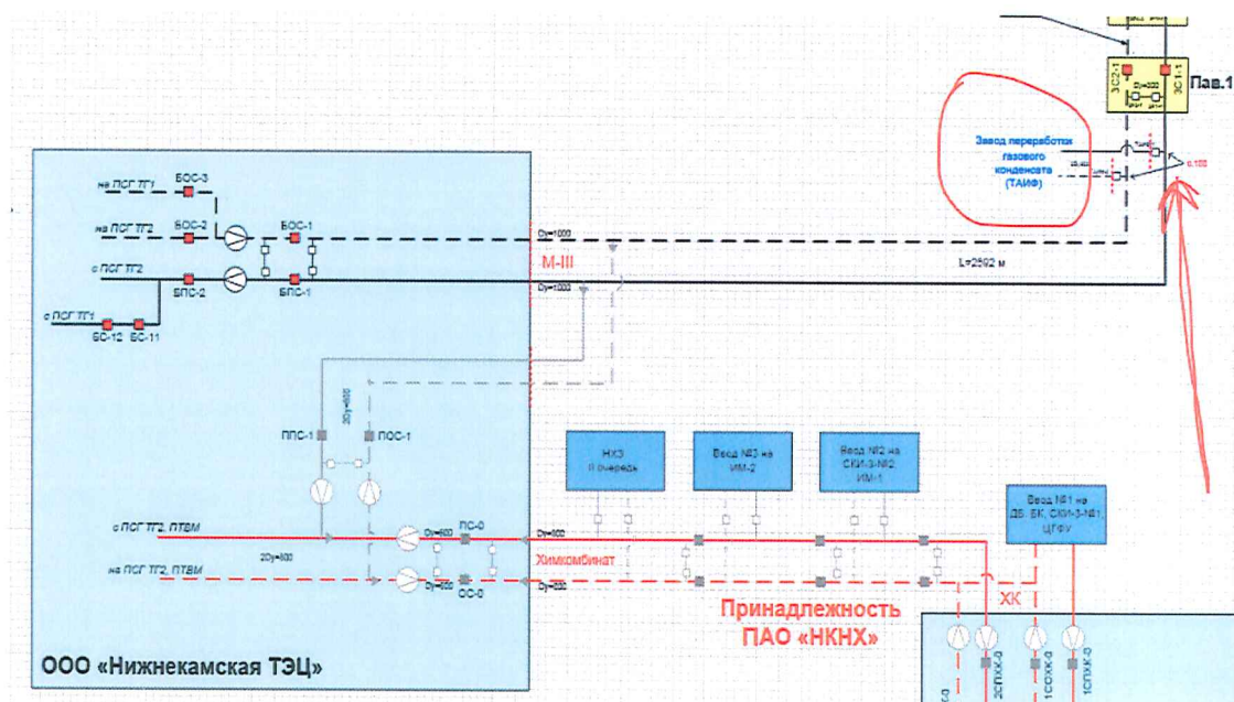
Рис. 1.3. Схема выдачи тепловой энергии в виде горячей воды от ООО «Нижнекамская ТЭЦ» (ППК-2)
